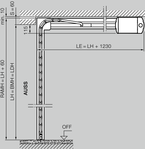
Størrelser for rulleport for montering under taket RollMatic OD
