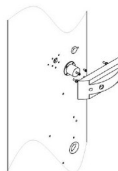
Elektromagnet
